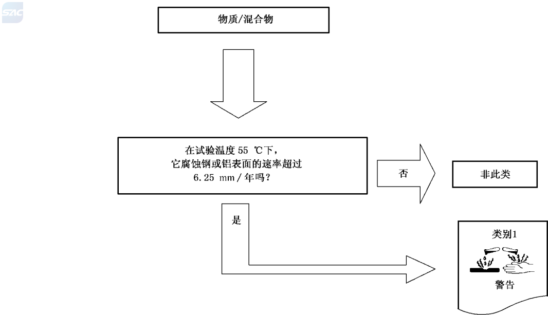
图 A.1 金属腐蚀物的判定逻辑
