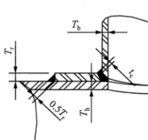
c) 带补强板的安放式焊接支管
