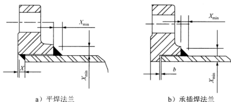
图 8.5.3-1 平焊法兰和承插焊法兰的角焊缝
