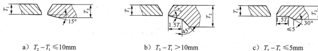
图 8.2.5-1 外壁齐平不同壁厚管道组成件坡口侧加工
