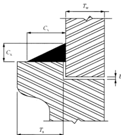
图 8.5.3-2 承插焊管件的角焊缝
