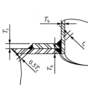
d) 带补强板的插入式焊接支管
