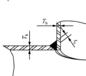
b) 插入式焊接支管
