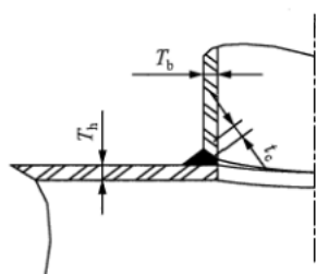
a) 安放式焊接支管
