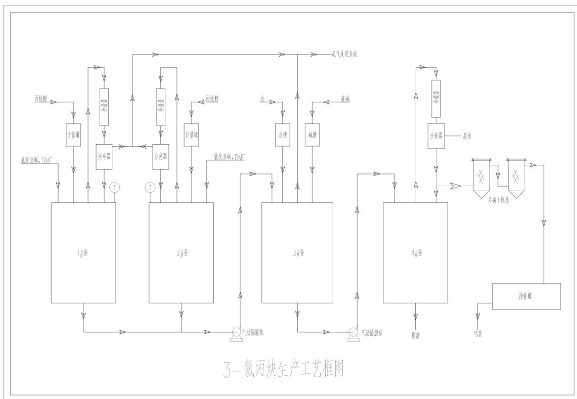
图3 3-氯丙炔生产工艺流程图示意图
