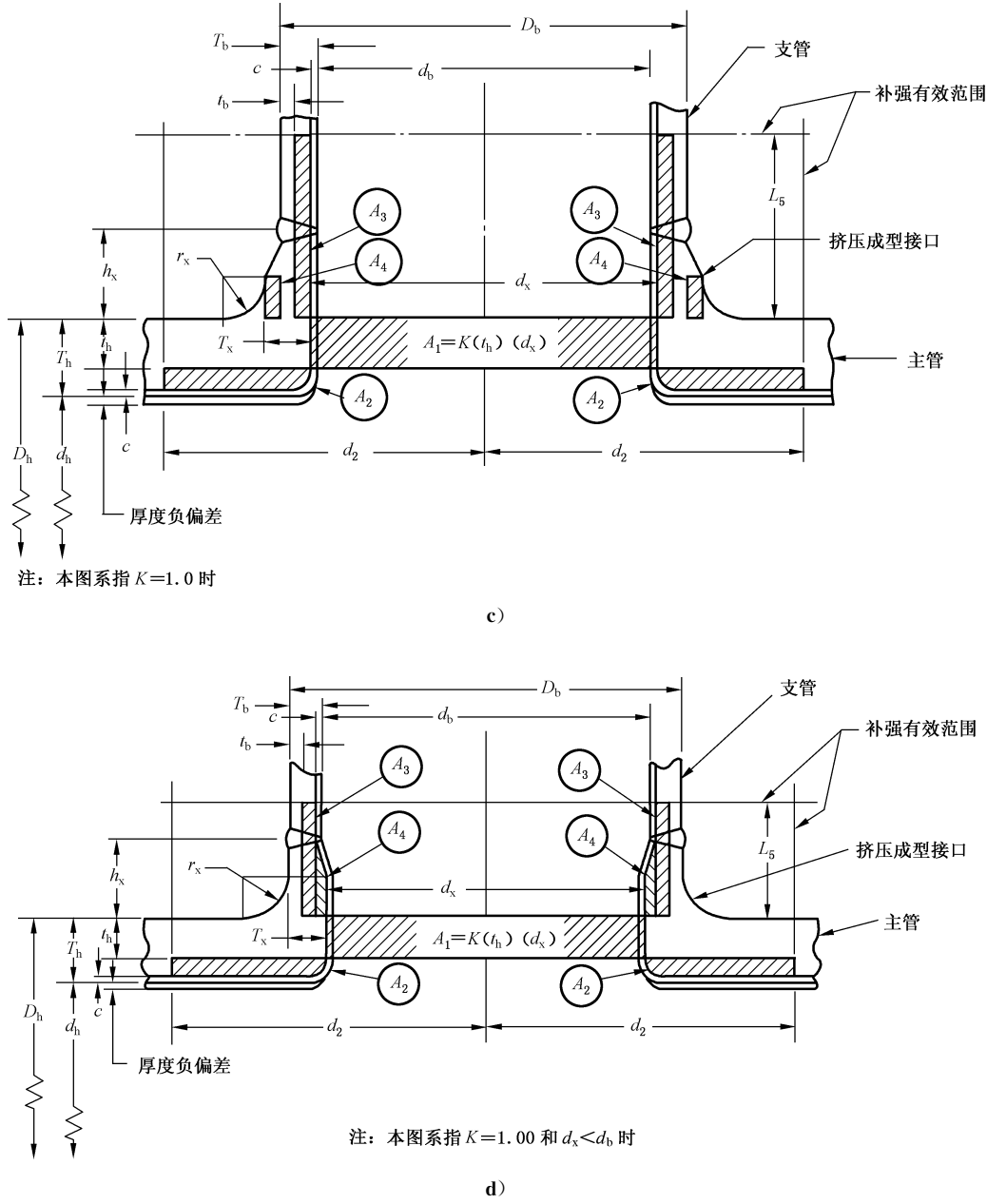
图 12 带挤压成型接口的支管连接（续）
