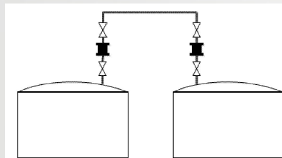
图 B-1 气相平衡管示意图 (连通的储罐为直接连通)
