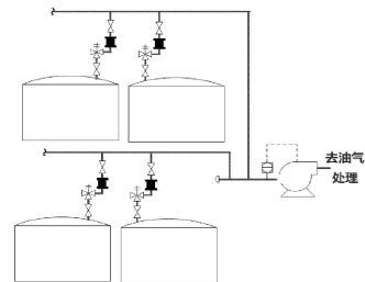
图 B-4 单呼阀方案示意图 (连通储罐不属于直接连通)
