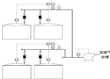
图 B-2 直接连通共用切断阀方案 (共用切断阀的一组储罐属于直接连通)
