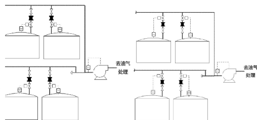
图 B-3 单罐单控示意图 (连通储罐不属于直接连通)
